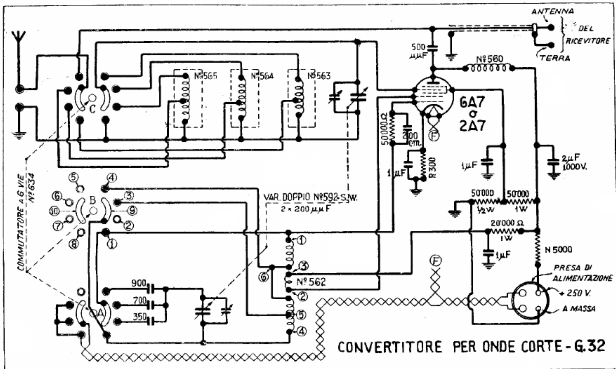
• Lo schema elettrico del G.32.
